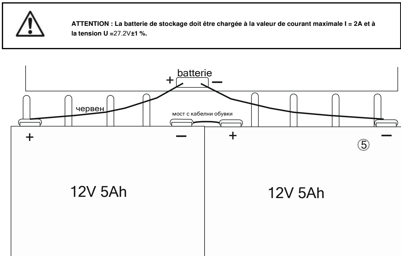
Fig. 7 Connexion des accumulateurs
